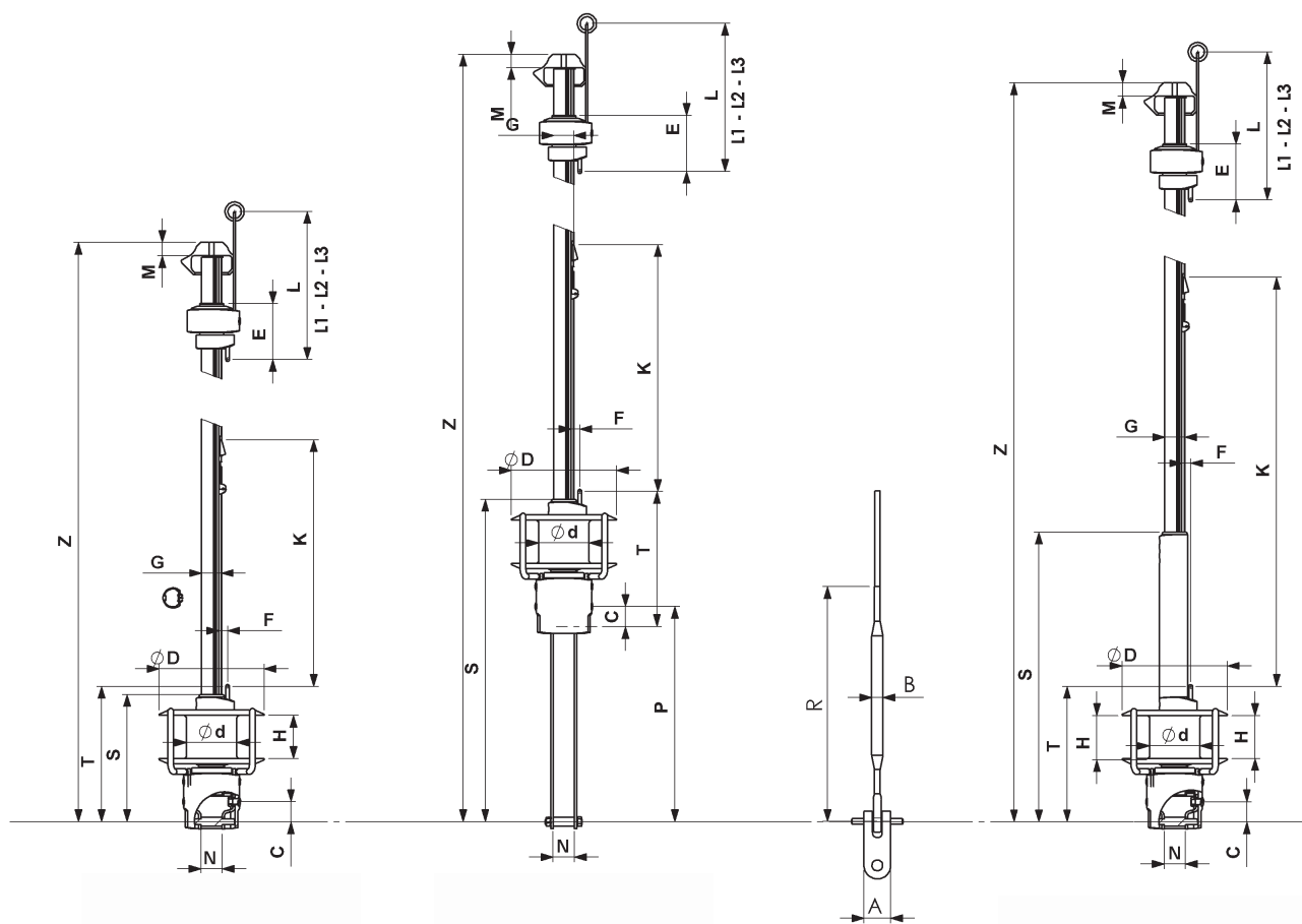
Lates longues (LL) Long link plates (LL)
